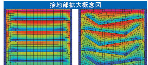
従来のサイプ(圧力が集中) リーフカットサイプ(圧力が分散)
